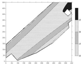
Рис. 10. Поверхность тренда второго порядка, подобранная по 72 точкам данных значений содержания клейковины в зерне, %
