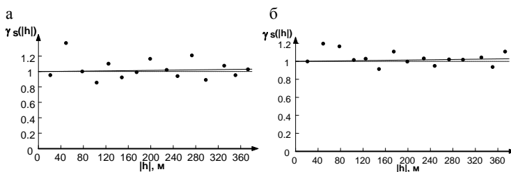
Рис. 9. Стандартизованные вариограммы для: а – содержание клейковины в зерне, %; б – показатель качества клейковины, ед. ИДК
