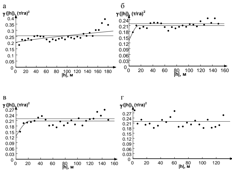
Рис. 13. Вариограммы для урожайности на контрольном участке: а – исходные данные, б – регрессионные остатки, все направления, в – направление 30^\circ , г – направление 120^\circ
