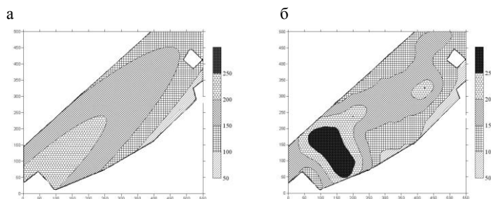
Рис. 8. Картограмма биомассы пшеницы в фазу цветения, г/м^2 в пределах поля, полученная с помощью: а – построения поверхности тренда второго порядка по 72 точкам данных значений; б – регрессионного кригинга
