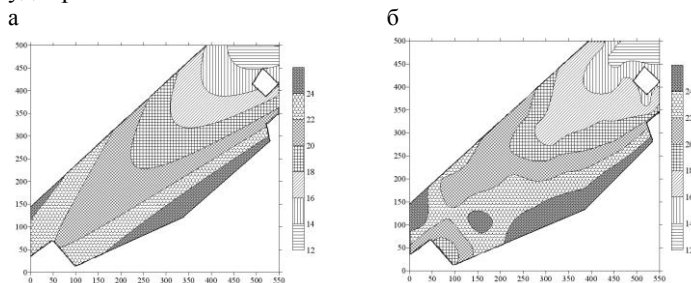
Рис. 6. Картограмма содержания доступного калия в почве, мг/100 г, полученная с помощью: а – построения поверхности тренда второго порядка по 72 точкам данных значений; б – регрессионного кригинга
