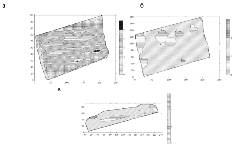
Рис. 12. Картограммы урожайности пшеницы (т/га), полученные с помощью регрессионного кригинга, а - вариант «точное земледелие», б – «хозяйственный вариант», в – контрольный вариант.
