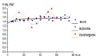
Рис. 3. Анизотропные вариограммы содержания органического углерода в пахотном слое
