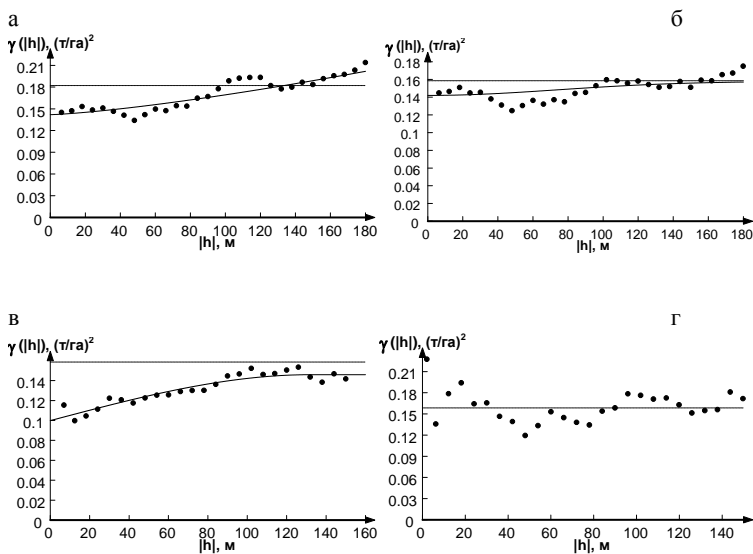
Рис. 14. Вариограммы для урожайности при «хозяйственном» варианте: а – исходные данные, б – регрессионные остатки, все направления, в - направление 30°, г - направление 120°
