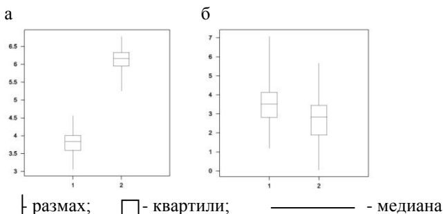
Рис. 1. Квартильное представление значений рН КCl (а) и содержания углерода С, % (б) для почв участков под лесом (1) и под пашней (2)
