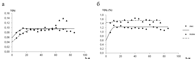
Рис. 2. Вариограммы для почвенных свойств (здесь и далее: точки – экспериментальные данные, линии – модель): а – рН, б – содержание органического углерода
